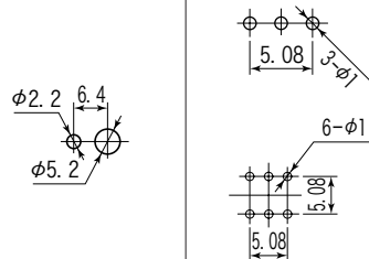
取付穴参考寸法 Mounting Hole
